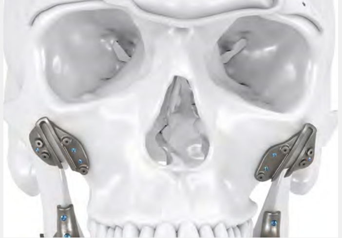
Guías para reducción cigomática De titanio de fabricación aditiva
